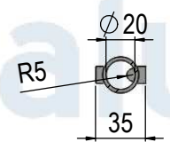
SECÃO A-A ESCALA 1 : 2
